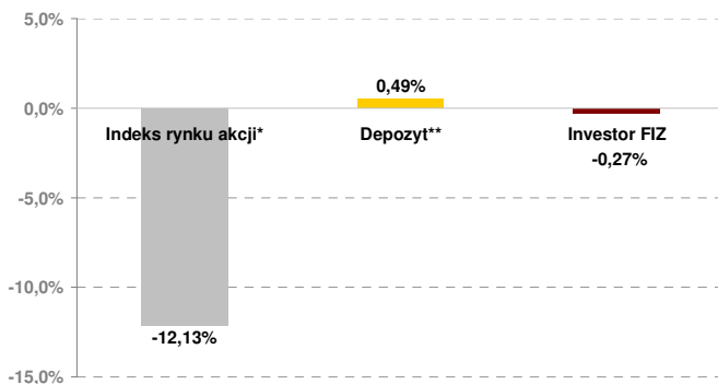
Stopa zwrotu 31.01.09 - 28.02.09 [%]
